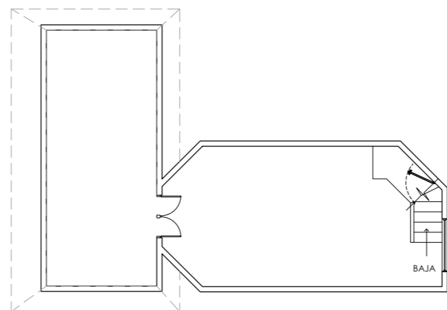
PLANTA PISO 2
